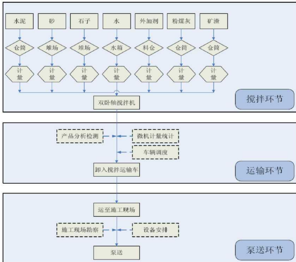
公司商品混凝土生产流程图
