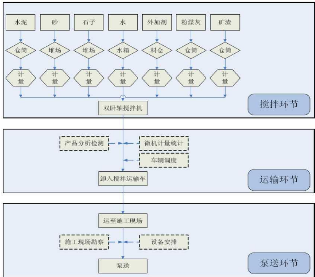
公司商品混凝土生产流程图
