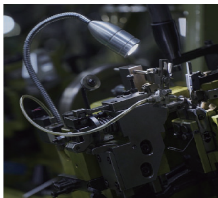
手鏈扣自動化加工設備
