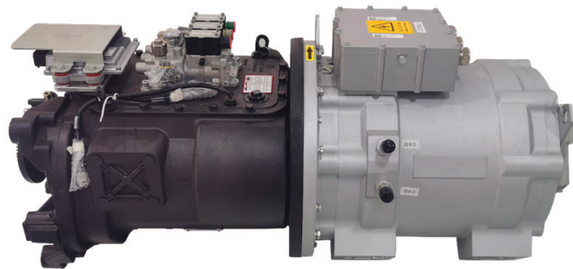
新能源牽引車的動力系統成套件
