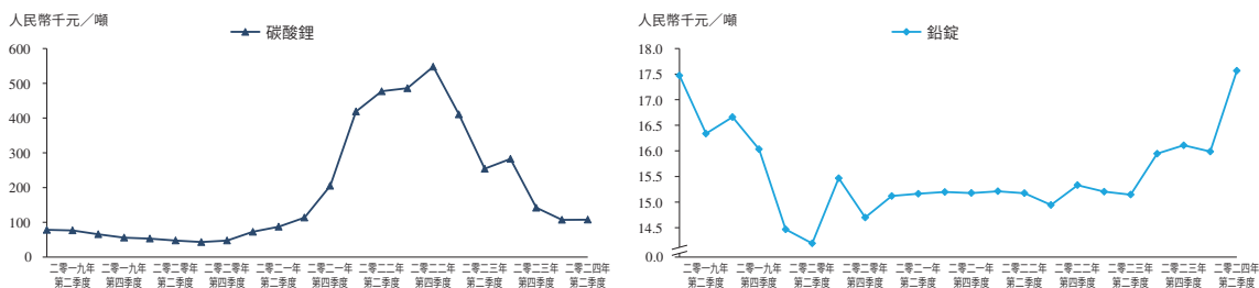
中國鋰離子電池和鉛酸電池主要原材料平均價格趨勢，二零一九年第一季度至二零二四年第二季度
