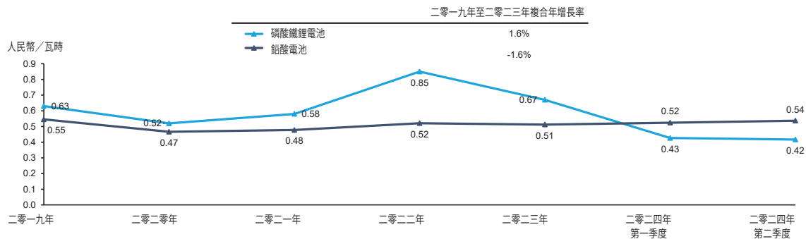
二零一九年至二零二四年第二季度磷酸鋰及鉛酸電池的平均價格(中國)
