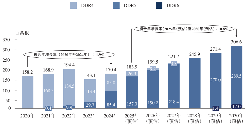
服務器內存模組出貨量，按內存顆粒代際拆分，全球，2020年至2030年（預估）
