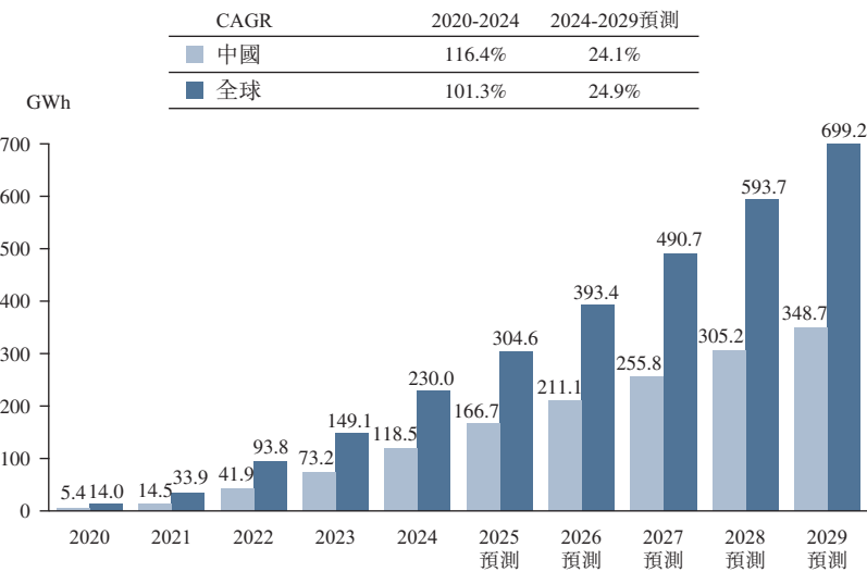
鋰離子電池儲能系統市場規模，以出貨量計，2020-2029預測
