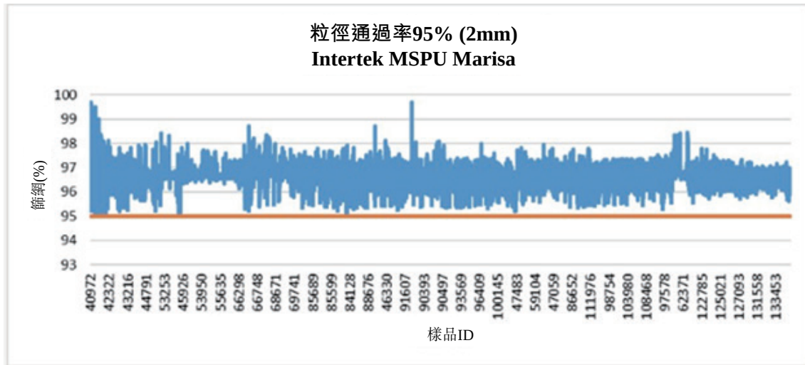
圖6-2篩選試驗—2毫米
