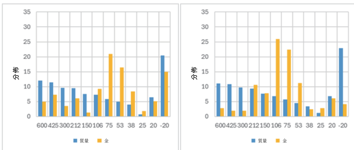
圖10-5 PETS 1及PETS 2樣品的粒度及金分佈
