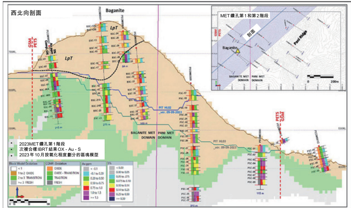
圖10-1堆浸試驗工作樣品選擇剖面圖1
