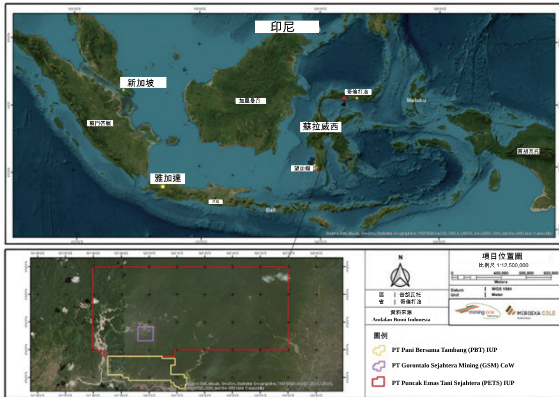
圖3-1 Pani金礦項目採礦許可證
