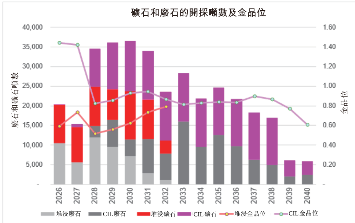
圖9-12 Pani年度採礦生產計劃
