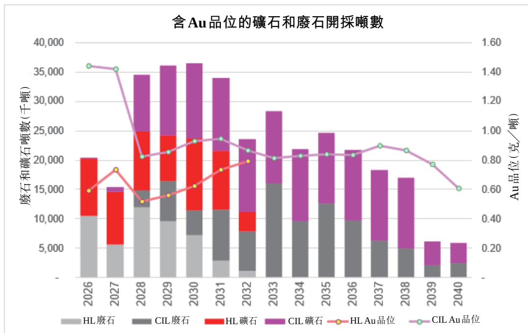
圖0-2年度採礦生產計劃
