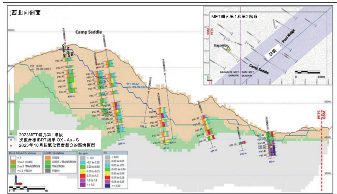
圖10-2堆浸試驗工作樣品選擇剖面圖2
