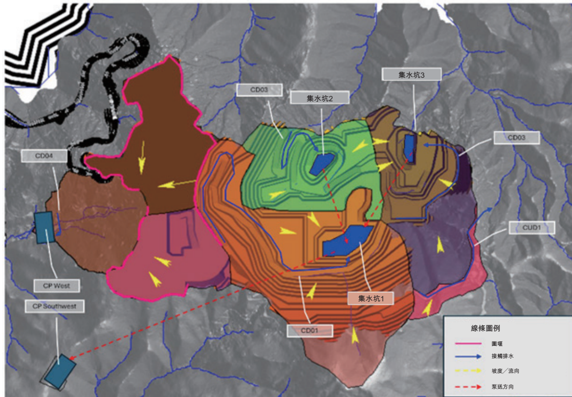
圖 9-1 礦坑水管理摘要 (WSP 2023)
