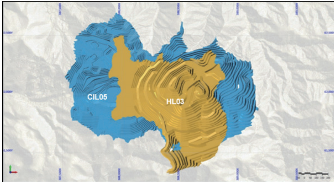
圖0-1 Pani礦坑設計概覽(顯示堆浸及炭浸區)
