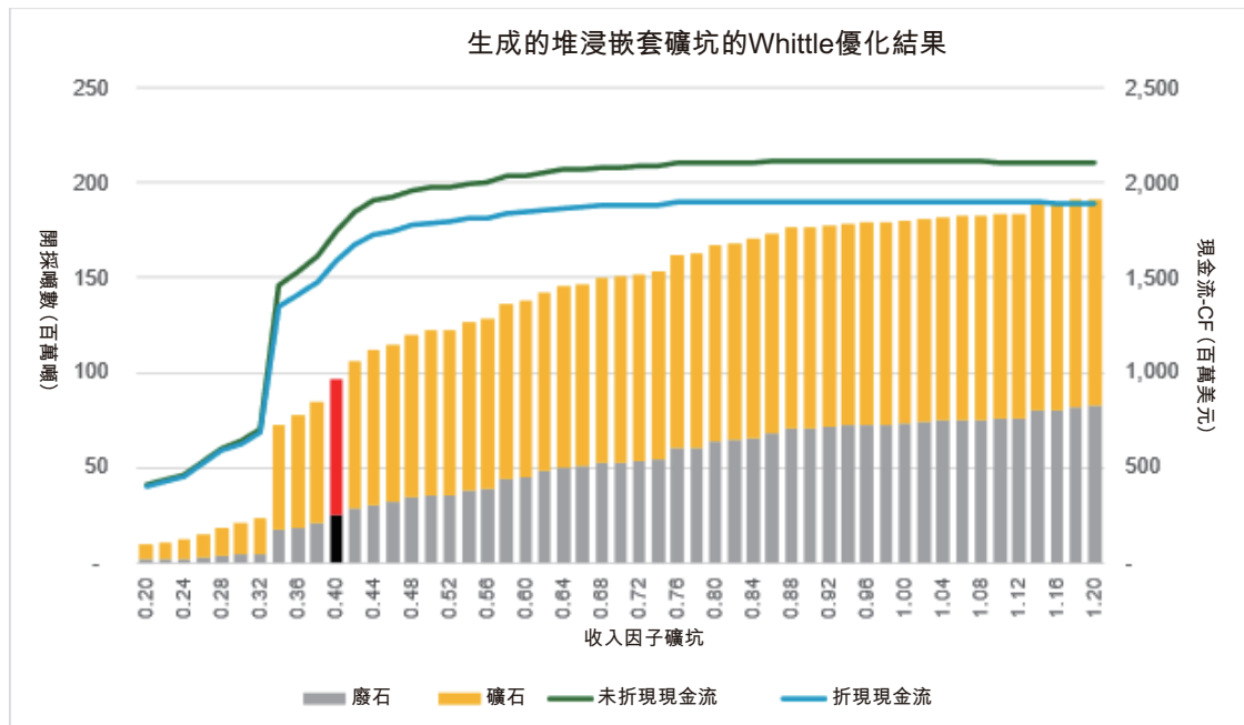
圖9-8限制於PETS IUP的堆浸優化逐坑圖
