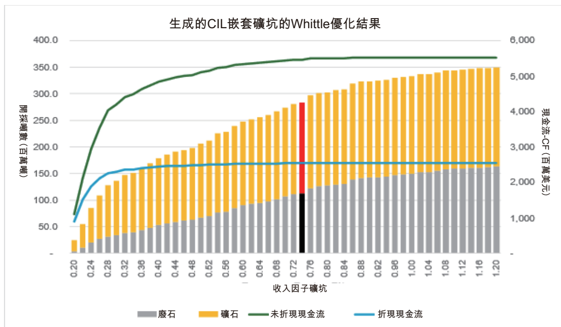
圖9-9無約束炭浸法優化逐坑圖
