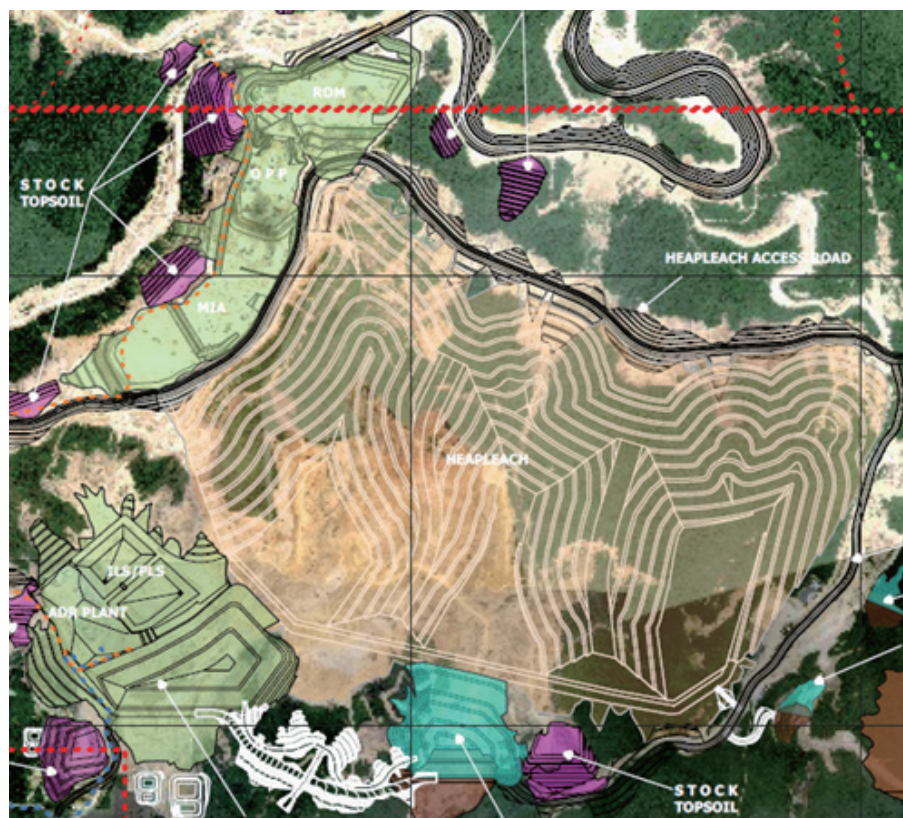
圖10-6堆浸設施及選廠位置
