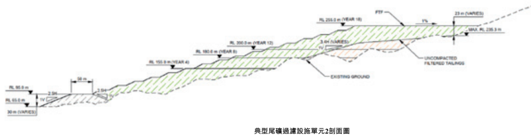
圖10-14尾礦過濾設施2號單元典型剖面
