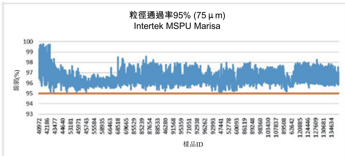
圖6-3篩選試驗—75微米
