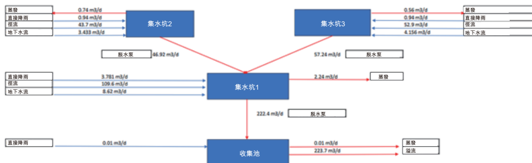
圖 9-2 水平衡流程圖 (WSP 2023)
