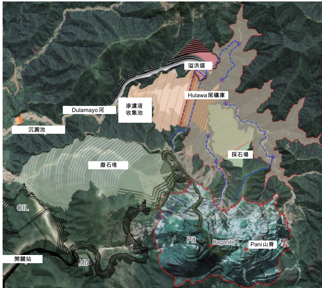
圖10-11 Hulawa尾礦庫設計佈置
