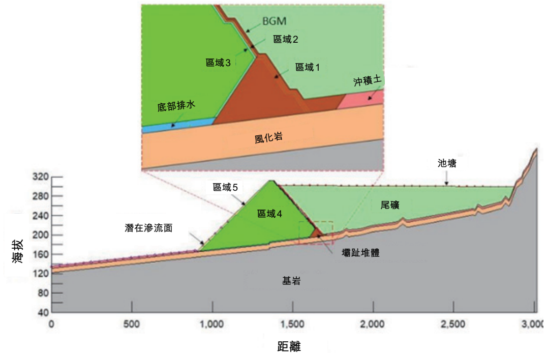
圖10-15尾礦庫滲流模型幾何形態及分層
