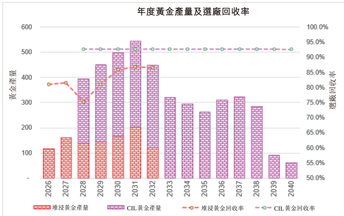
圖9-14 年度黃金產量及選廠回收率
