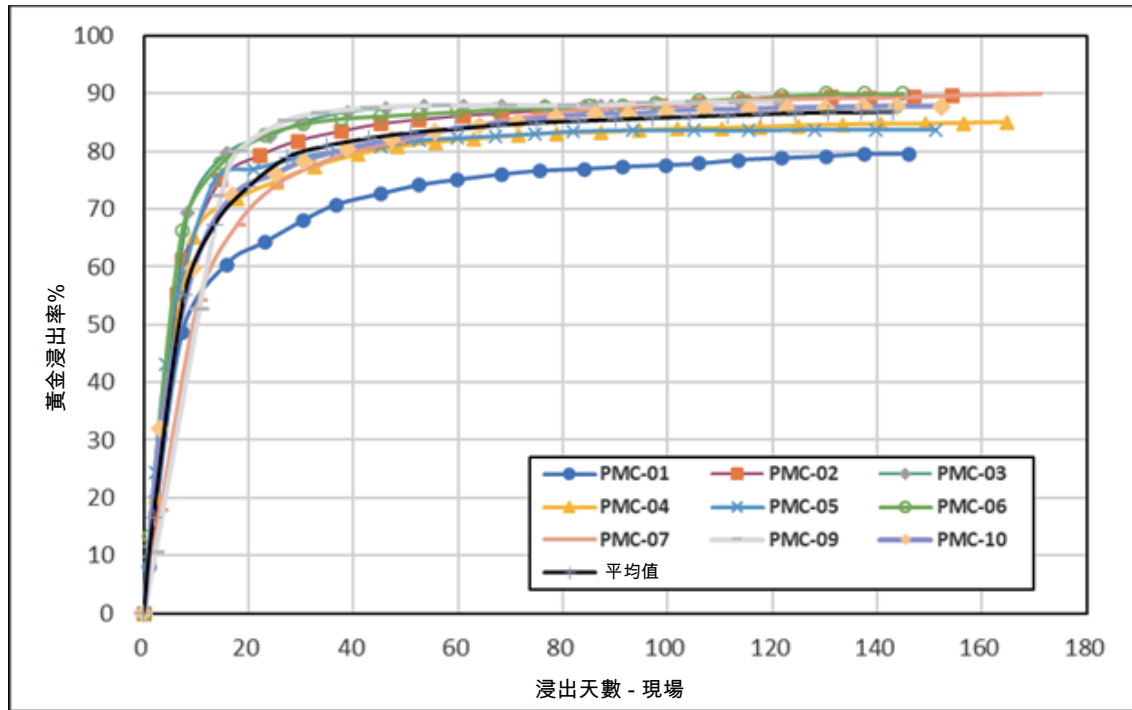
圖 10-4 根據 2024 年 5 月更新結果得出的 PETS 預計現場浸出曲線
