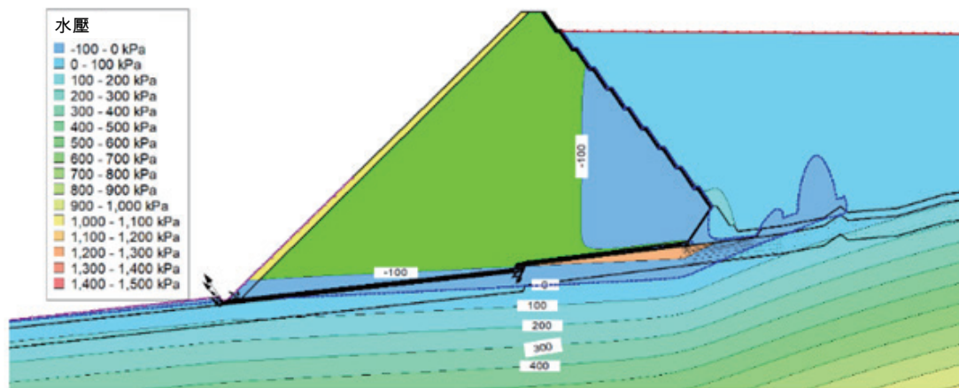
圖10-16尾礦庫滲流模擬孔隙壓力
