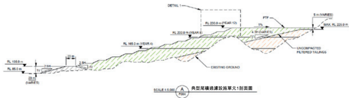
圖10-13尾礦過濾設施1號單元典型剖面
