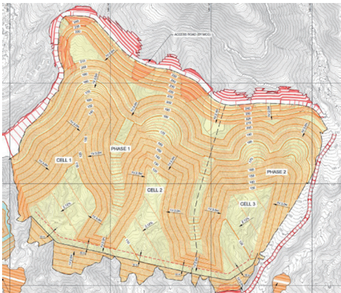
圖10-10堆浸設施建議施工階段
