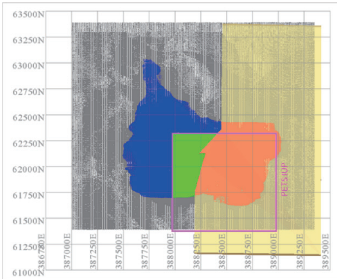
圖9-7用於礦山規劃的選礦區
