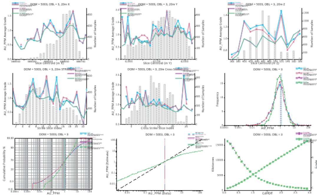
圖7-12金一域5003_3 (5303)的組合樣(粉紅色)、去叢聚組合樣(藍色)與塊體(青色)、信息塊體(綠色)的帶狀圖
