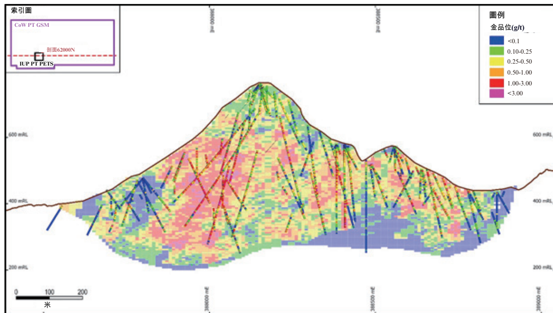
圖7-9代表性東西剖面(北坐標62000米)
