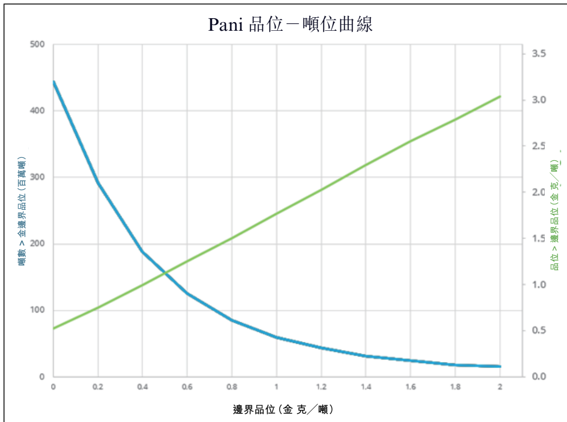
圖 7-14 Pani 金礦品位－噸位曲線
