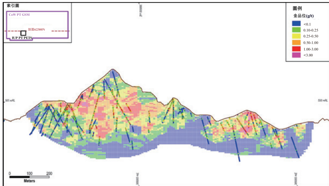
圖 7-10 代表性東西剖面(北坐標 62300 米)
