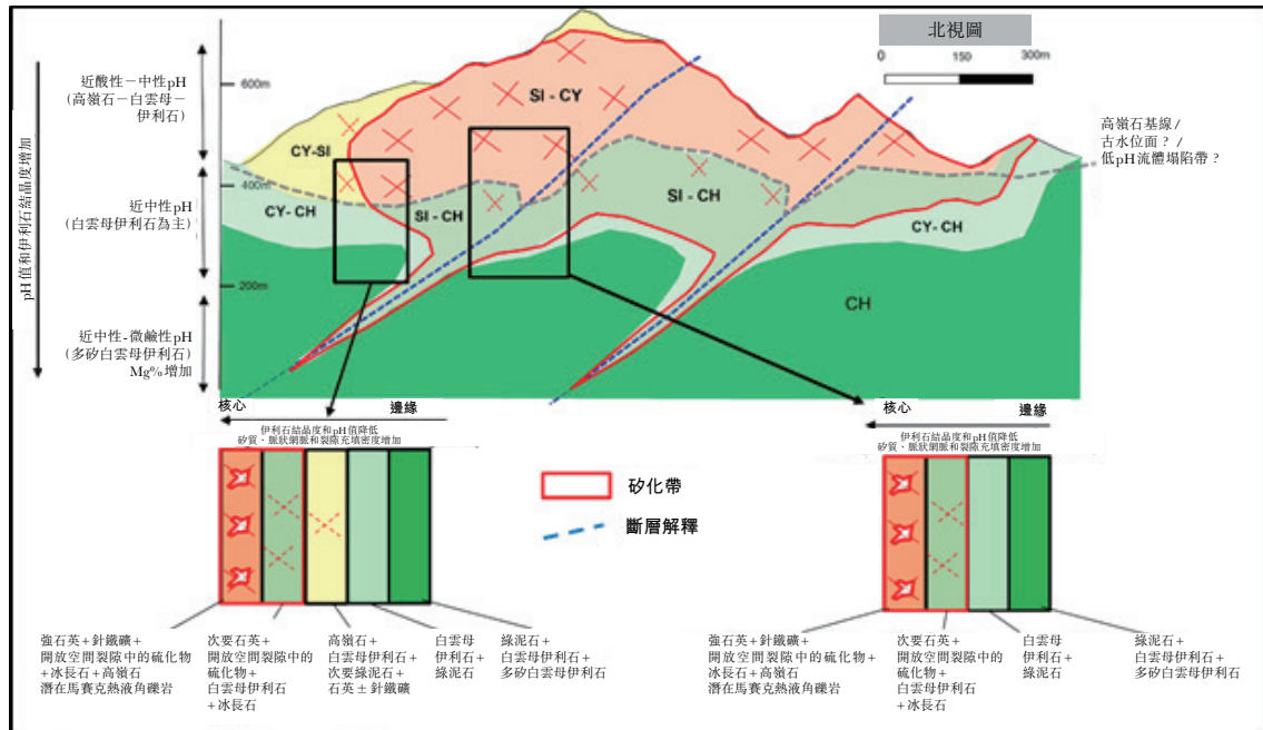
圖 5-5 Pani 蝕變簡化模型
