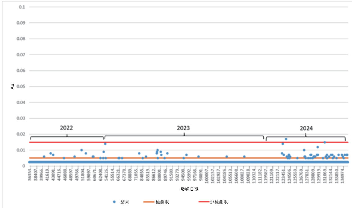
圖 6-5 黃金空白樣表現圖表
