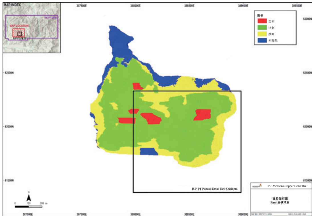
圖 7-13 Pani 資源量分類圖
