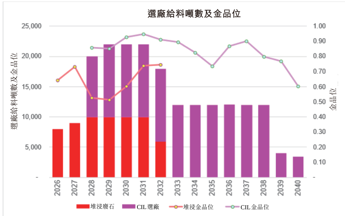
圖9-13 Pani 年度選礦給料計劃
