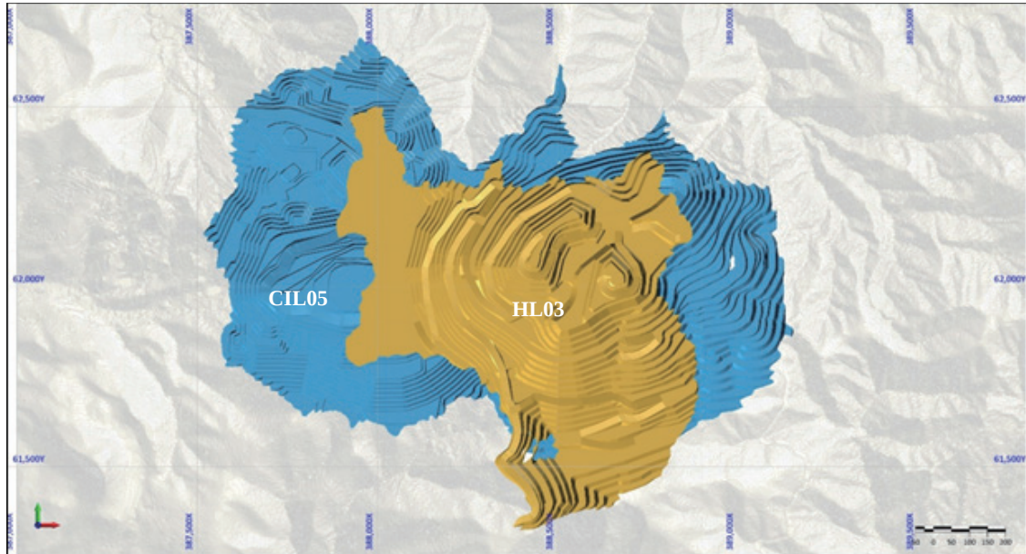
圖9-11 最終堆浸及炭浸法礦坑設計平面圖
