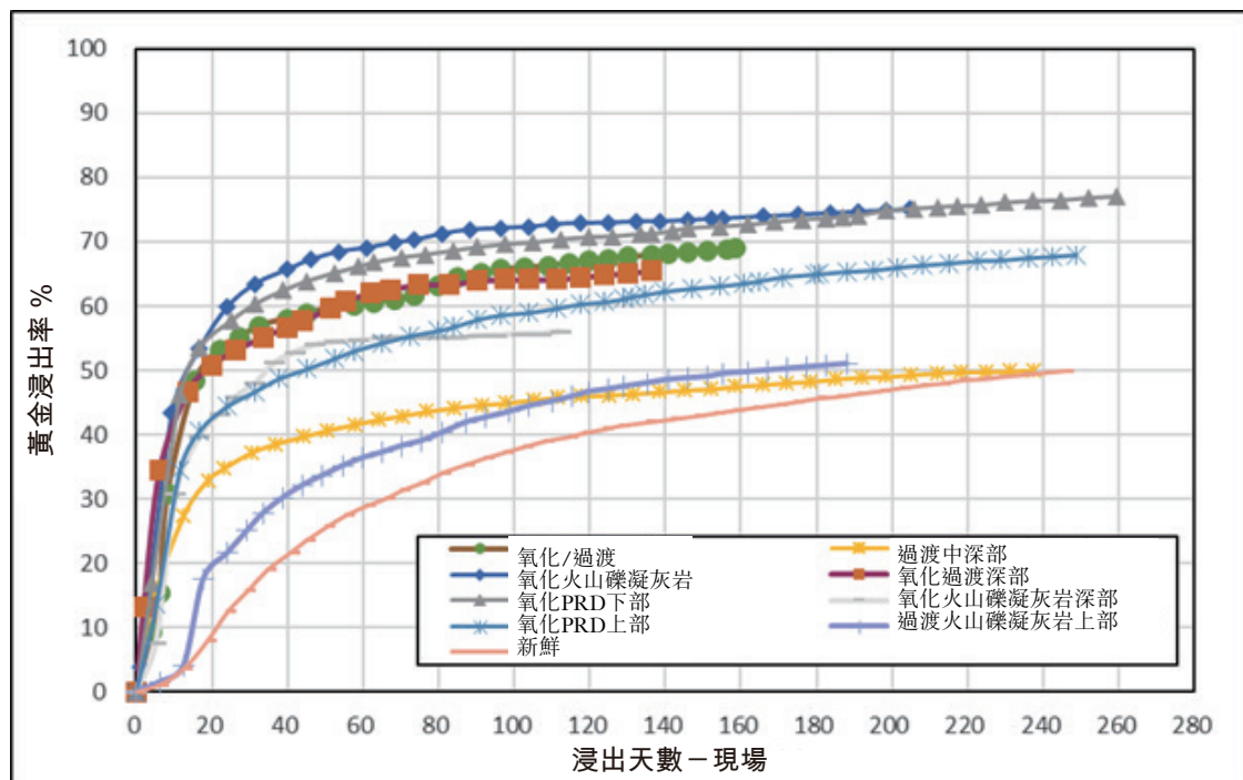
圖10-3 根據2024年5月更新結果得出的Baganite預計現場浸出曲線
