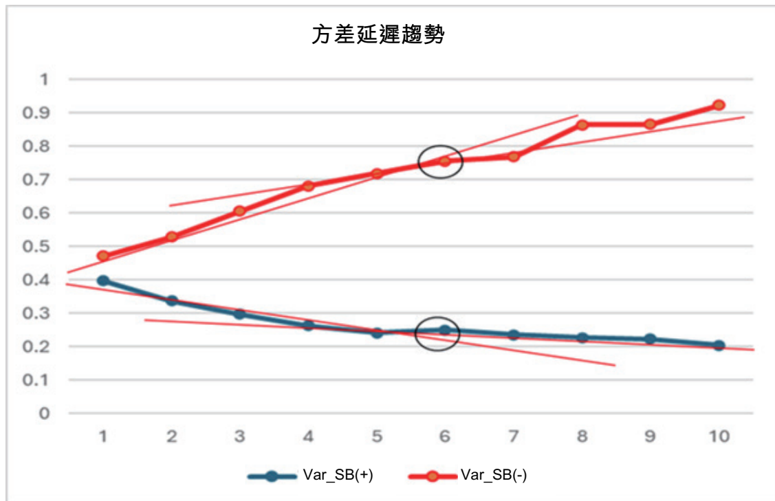
圖7-3來自高品位域的方差滯後趨勢(紅色為朝向，藍色為遠離)
