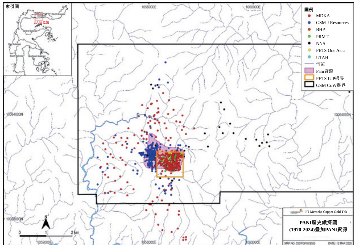
圖6-1 Pani鑽探工程(1970年至2024年)
