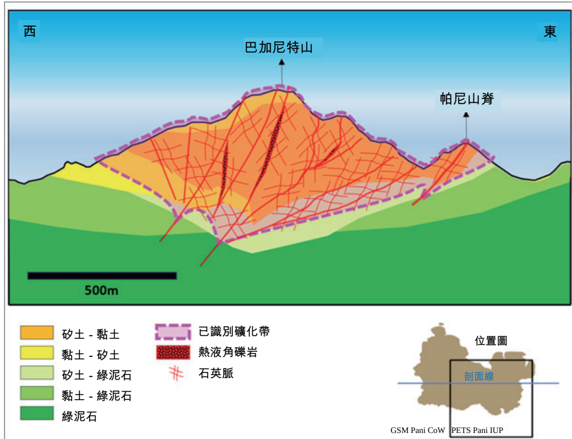
圖5-4 Pani地質與礦化帶概念剖面圖
