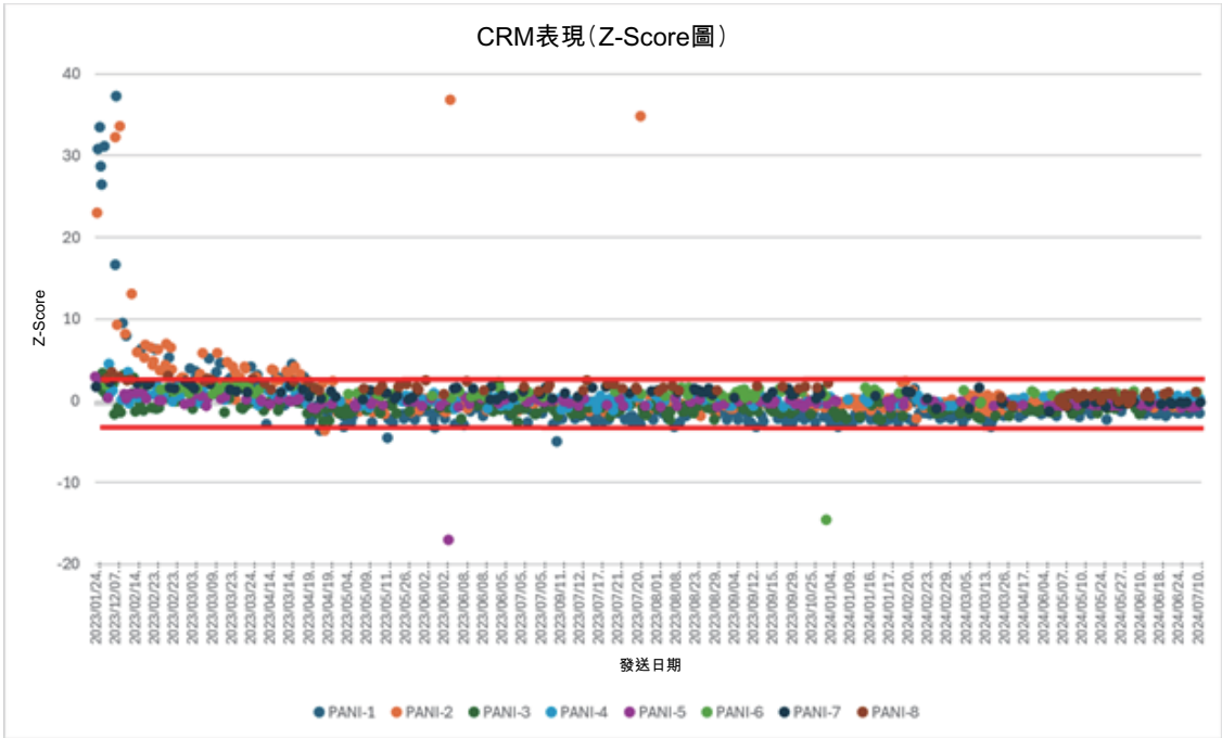
圖 6-4 基質匹配表現 (Z-Score)
