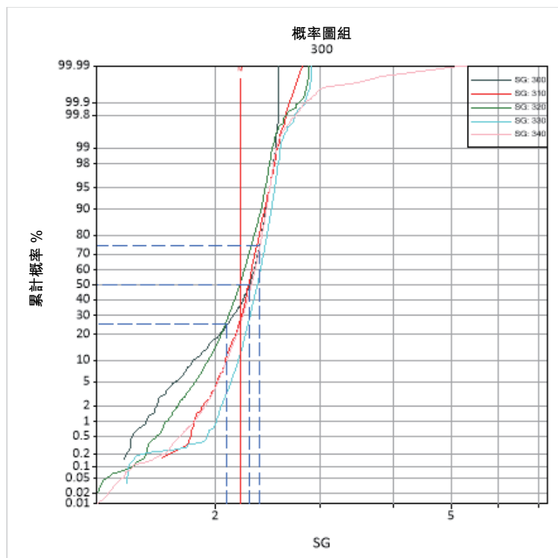
圖 7-5 蝕變與密度的對數概率圖
