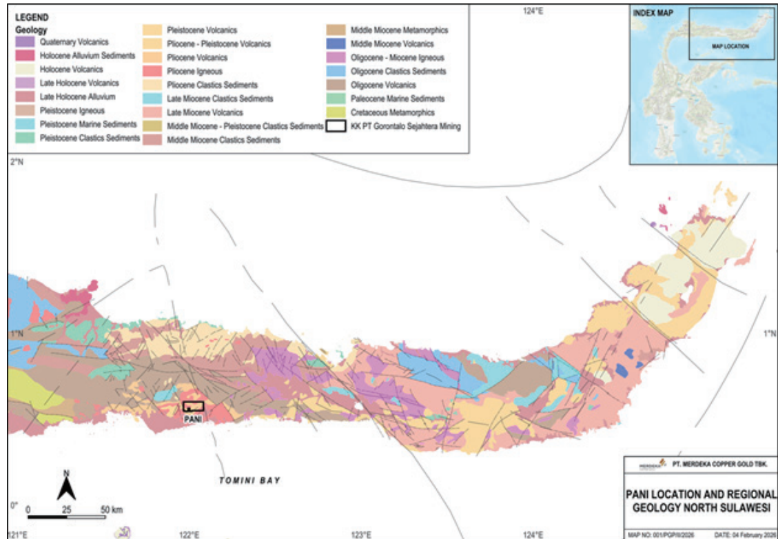
圖5-1 Pani區域構造背景
