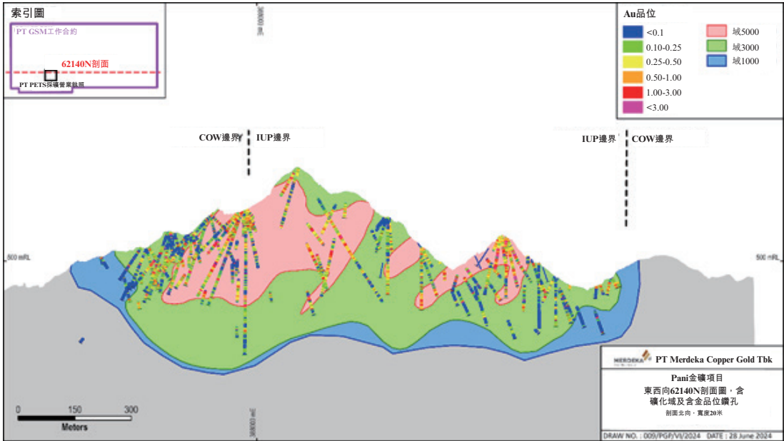
圖 7-1 Pani 原生資源域於北坐標 62140 米剖面
