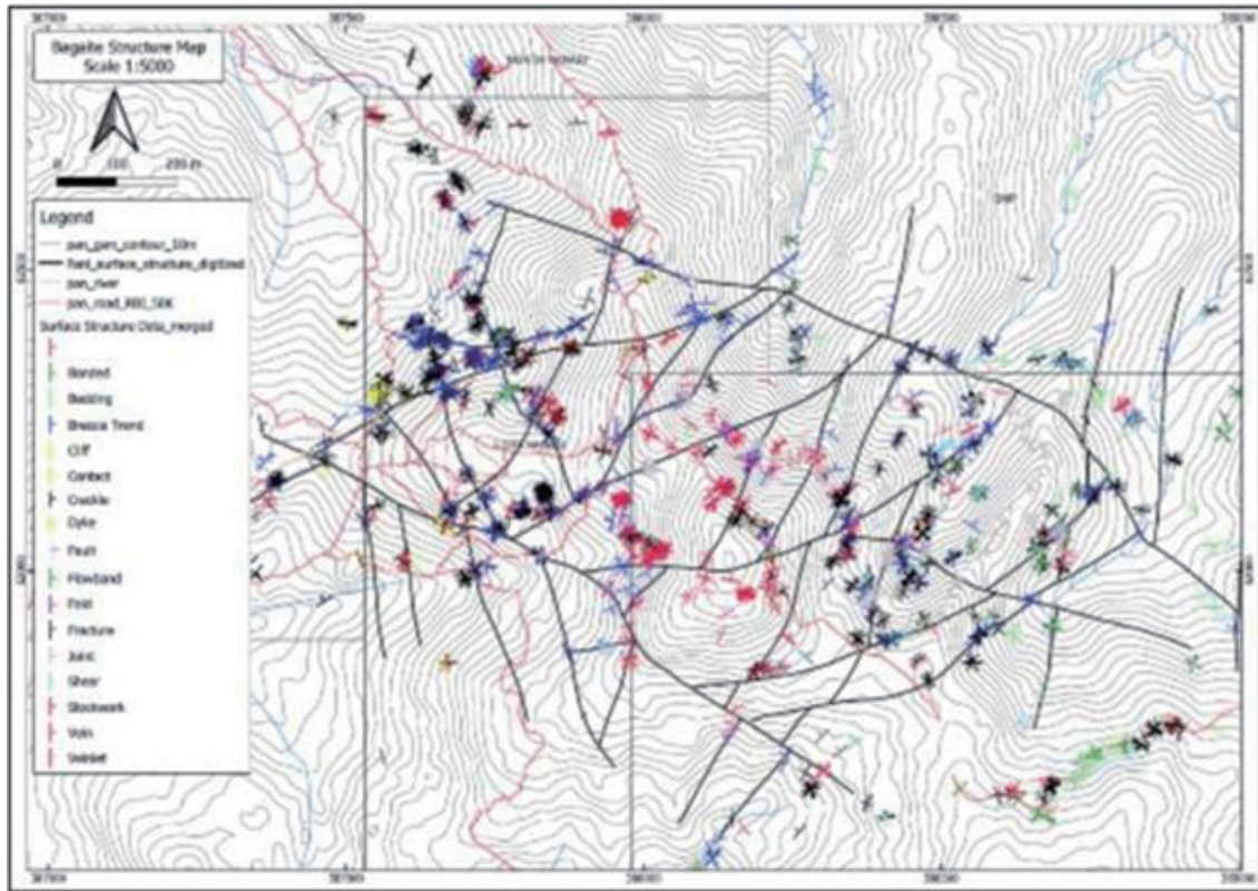
圖9-1 Pani礦床區域主要斷層(MCU，2023)
