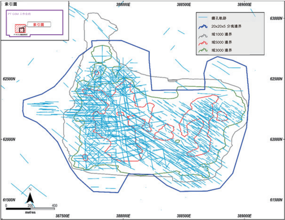
圖 7-4 鑽孔分佈(藍線為 20 × 20 × 5 格網塊體邊界)
