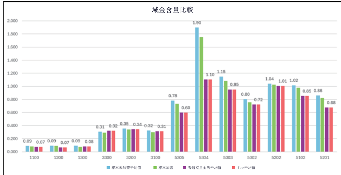
圖7-8域比較樣品與估算
