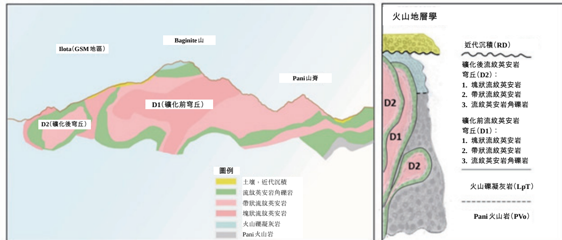
圖 5-2 Iloa– Baganite– Pani 山脊概念模型
