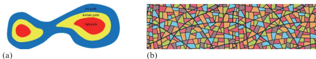
圖 7-6 (a) 擴散型礦化系統及 (b) 鑲嵌型礦化系統示例
