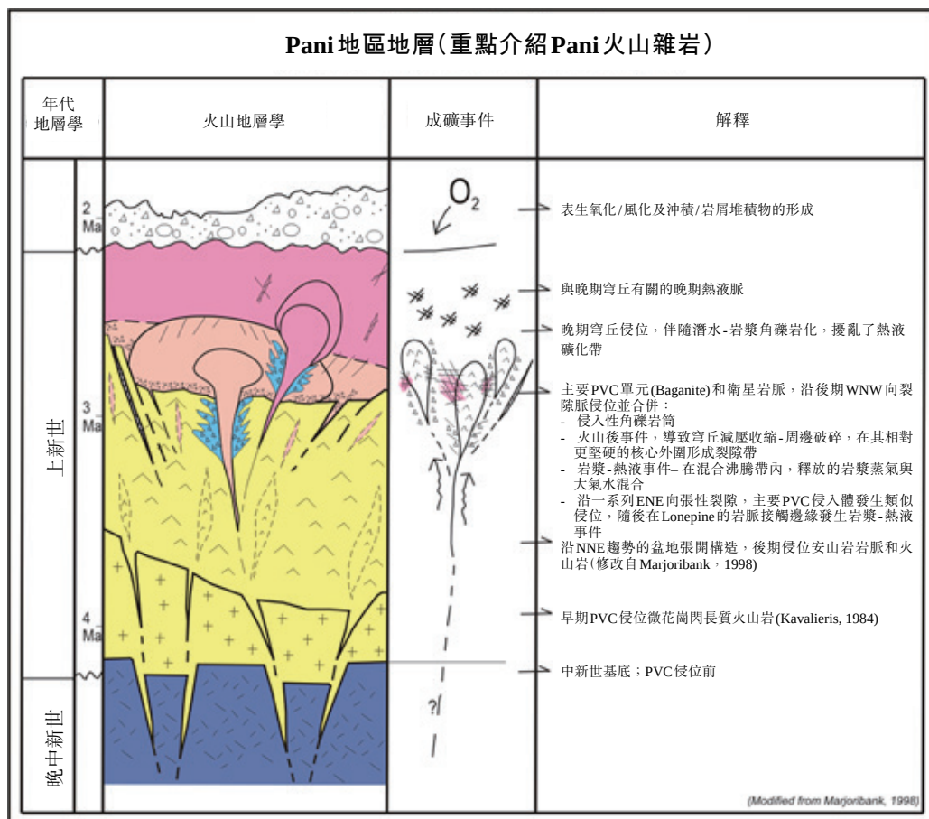
圖 5-3 Pani 地區地層
