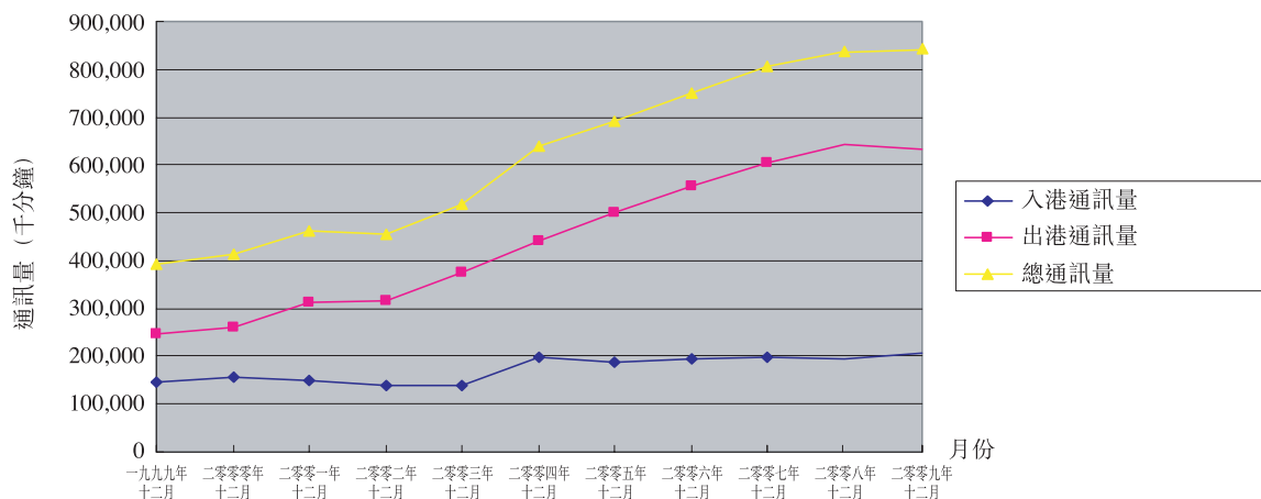
一九九九年十二月至二零零九年十二月香港ETS總通訊量
