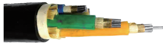
特種鋁電纜
