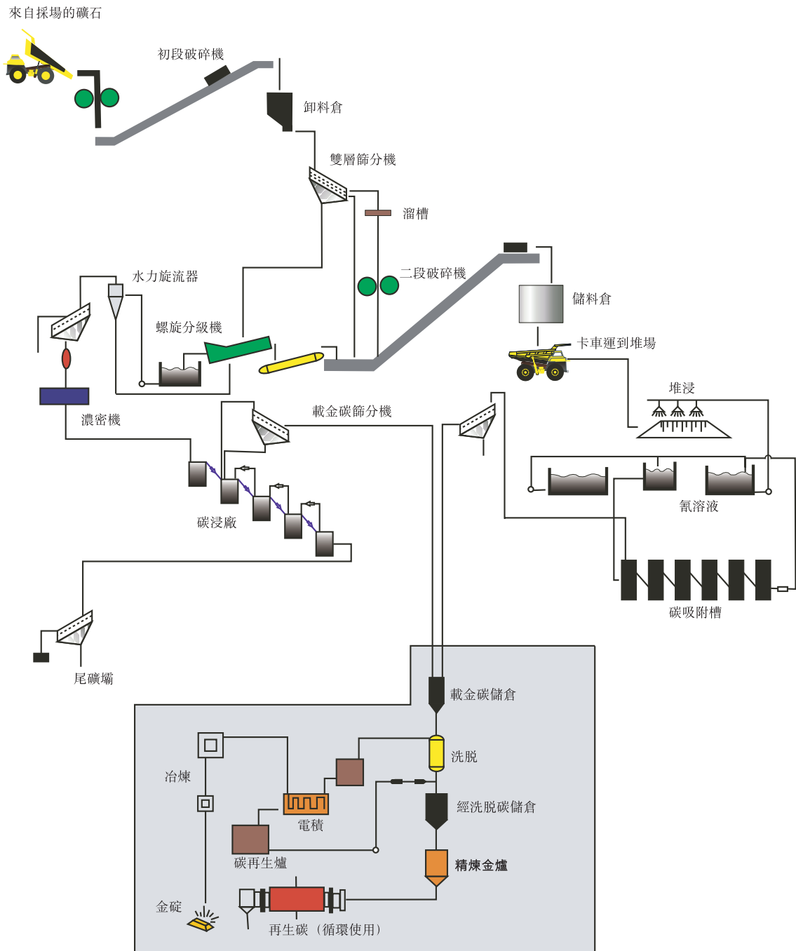
圖 8.1 紫金山－金礦選冶工藝流程圖
