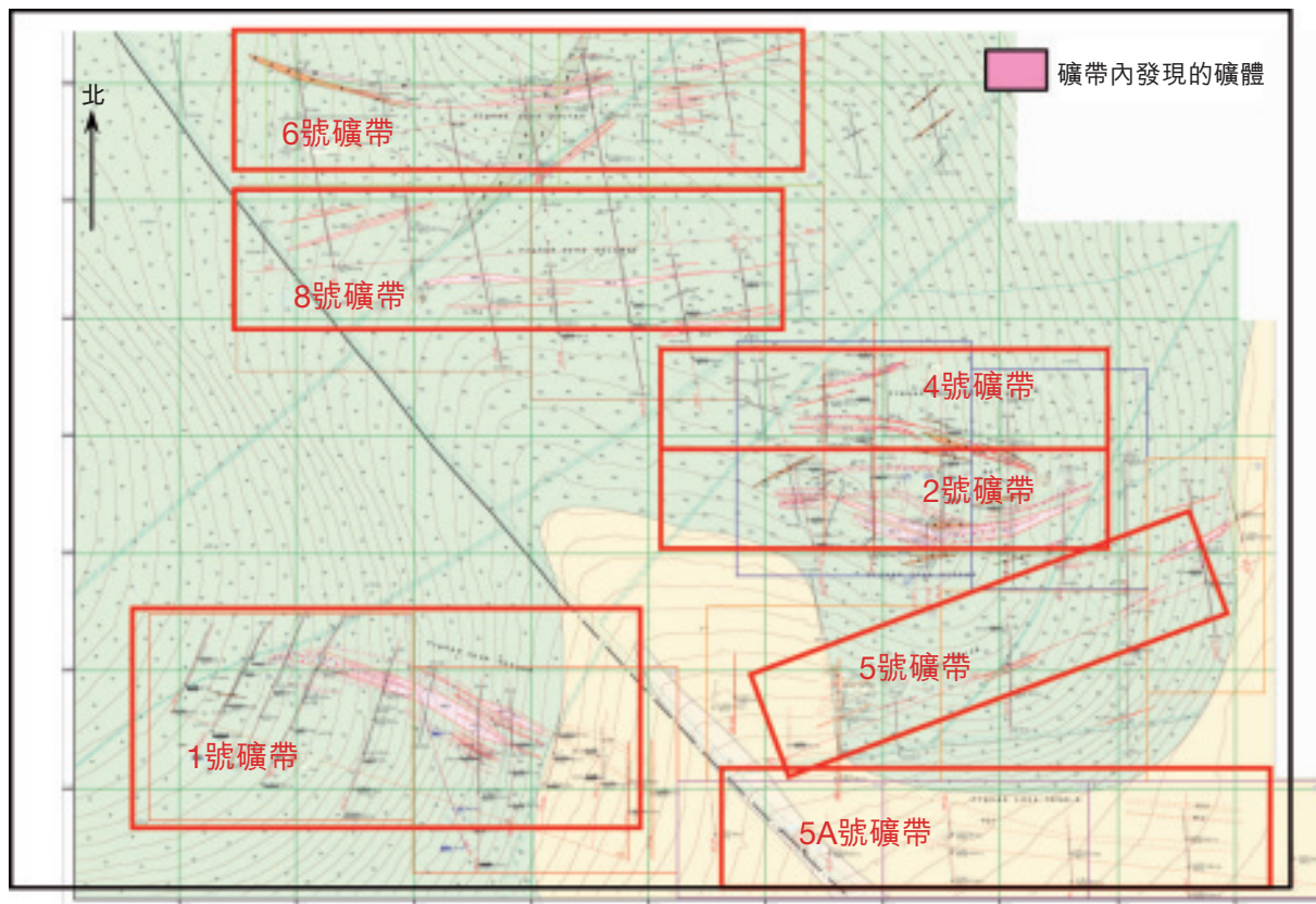
圖2.10 : Saikta 礦床的礦帶位置
