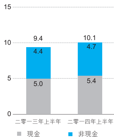
甘其毛都的經營現金成本總額 1 (美元/噸)
