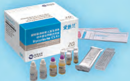
解脲脲原體和人型支原體 培養鑒定藥敏試劑
