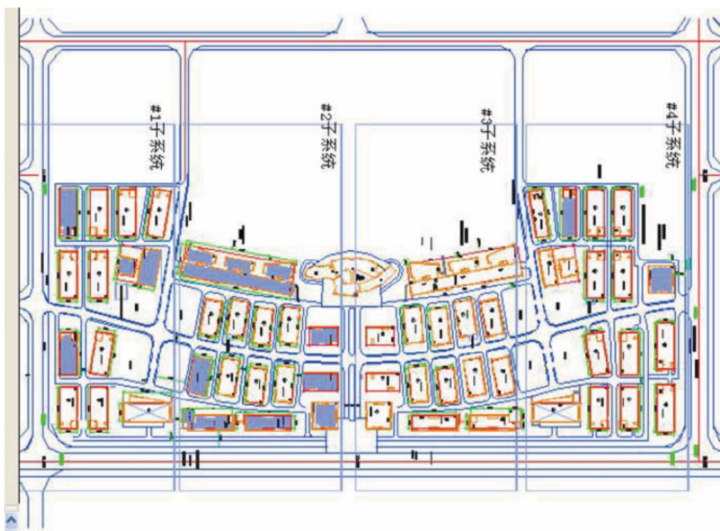
圖6.1發電站平面規劃圖 — 鎮江光伏設施
