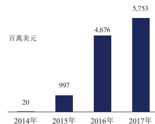
2014年至2017年Opdivo的全球銷售收入
