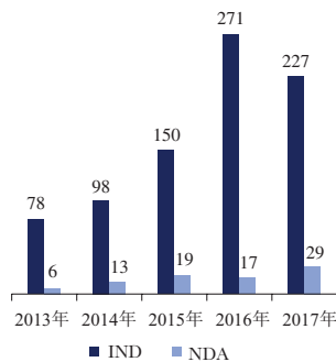
藥品審評中心批准的生物藥物IND 申請及NDA（2013年至2017年）
