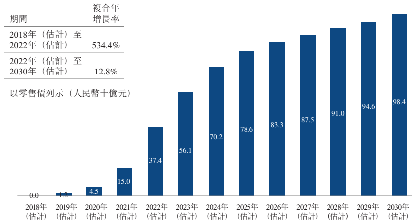
中國PD-1及PD-L1抗體的市場規模預測（2018年（估計）至2030年（估計））
