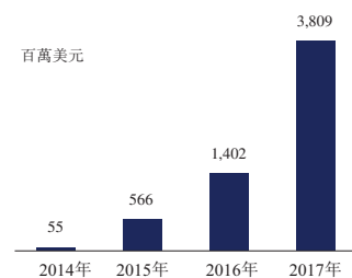
2014年至2017年Keytruda的全球銷售收入
