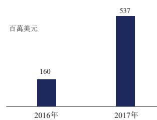
PD-L1單抗的銷售收入（2016年至2017年）
