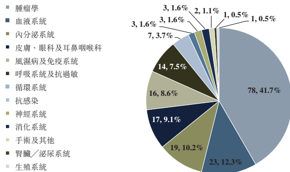
2017年治療領域批准的 生物藥物IND申請
