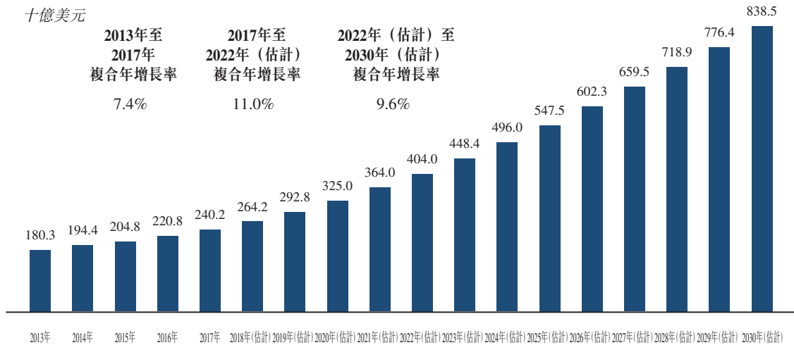
全球生物藥物市場的市場規模（2013年至2030年（估計））
