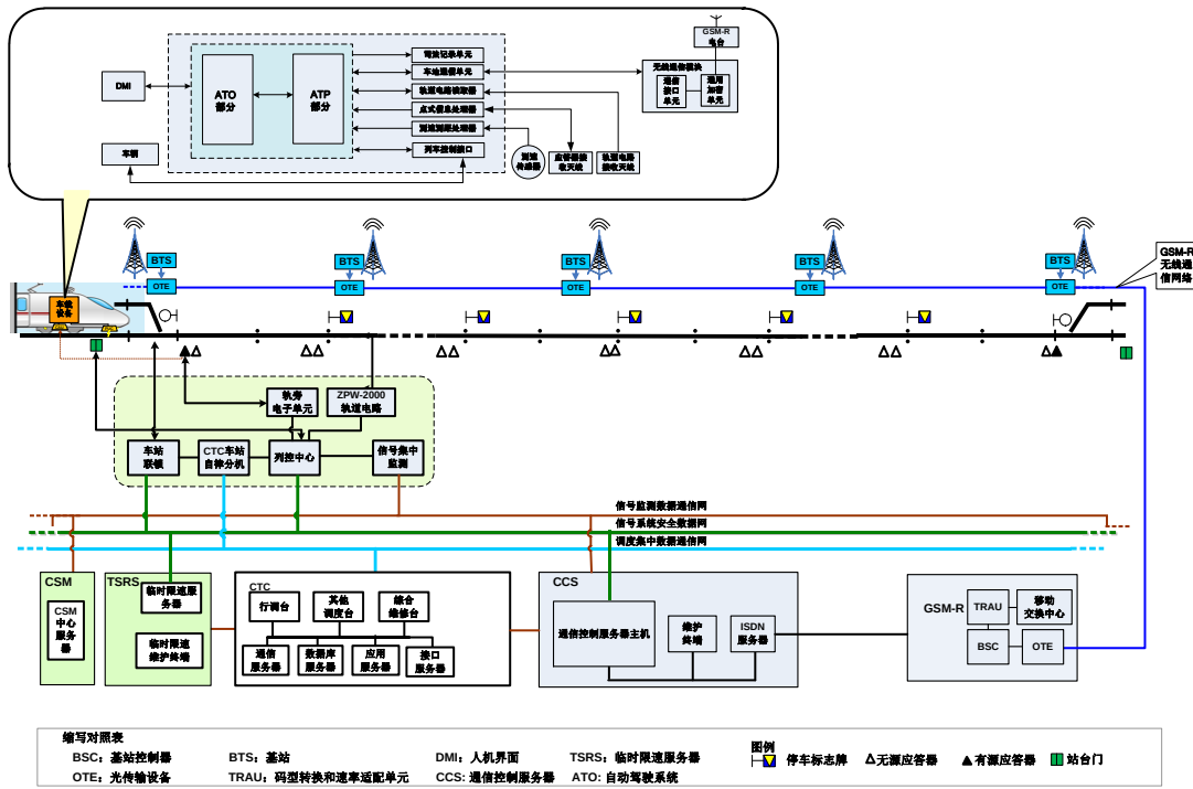
CTCS-2+ATO 系统示意图
