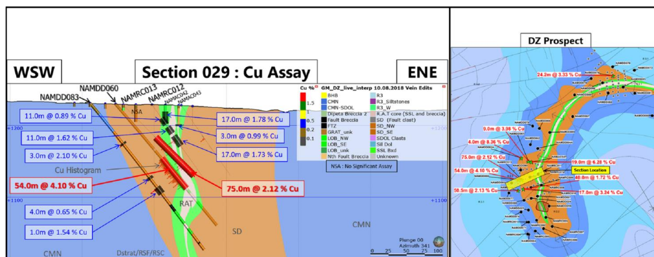
圖 12：DZ 勘探區典型鑽孔剖面圖。
