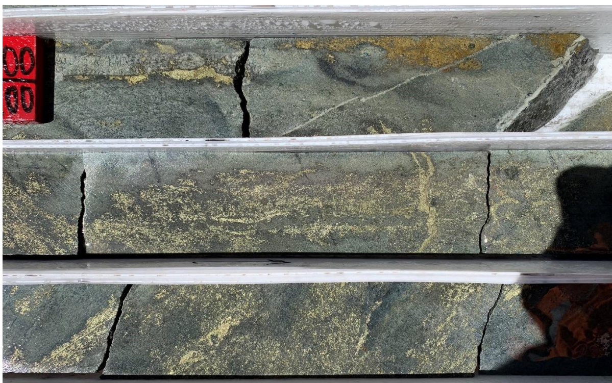
圖 6：5 所述的矽卡岩型浸染狀黃銅礦化特寫圖。
