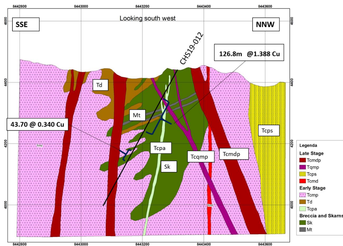
圖 4：鑽孔 CHS19-012 地質剖面圖，鑽孔位置見圖 2。
