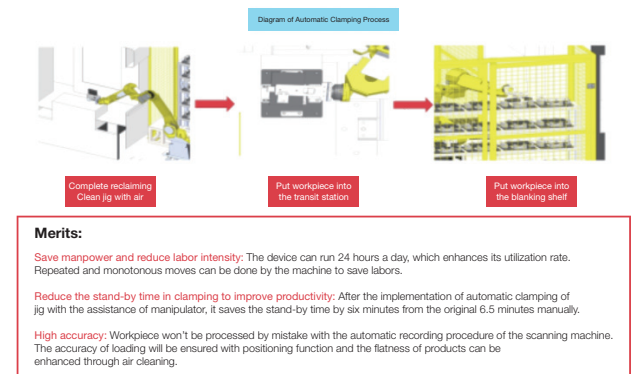
圖2：自動裝夾工序示意
