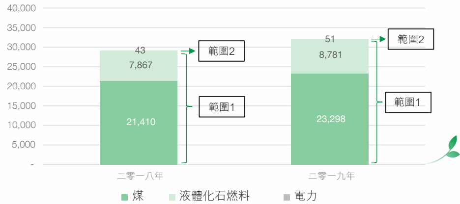
按燃料類型劃分的溫室氣體排放(噸二氧化碳當量)
