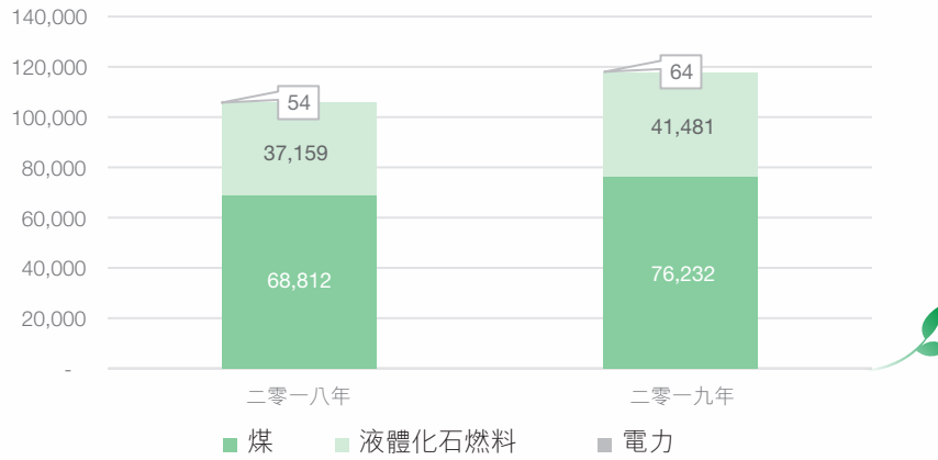
按燃料類型劃分的能源使用(兆瓦時)
