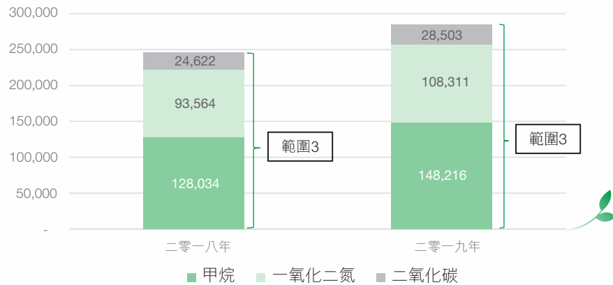
牧場上的溫室氣體排放按氣體類型劃分(噸，噸二氧化碳當量)
