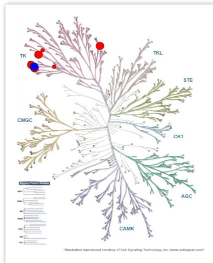
Zanubrutinib
