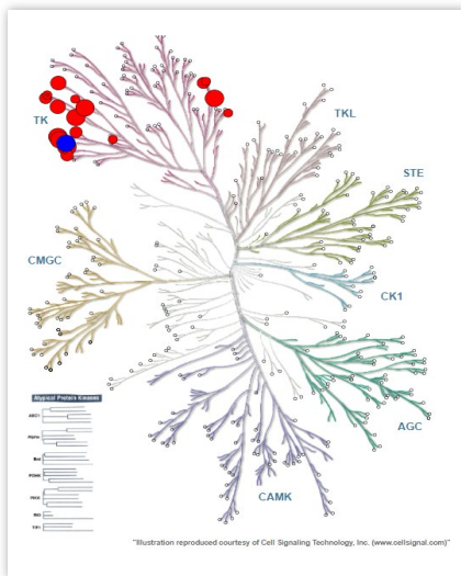
Ibrutinib
