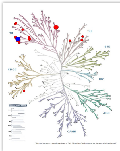
Acalabrutinib
