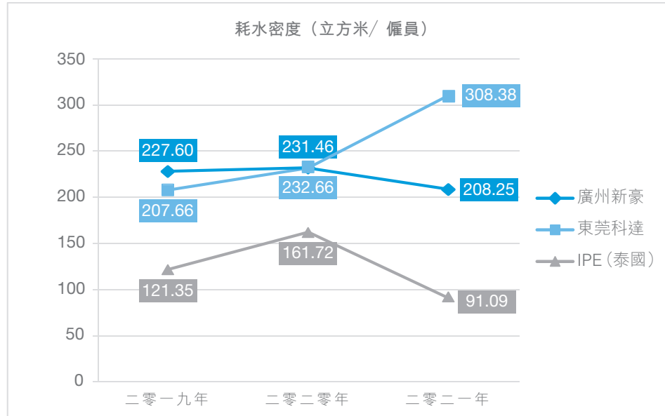
圖4二零一九年至二零二一年耗水密度
