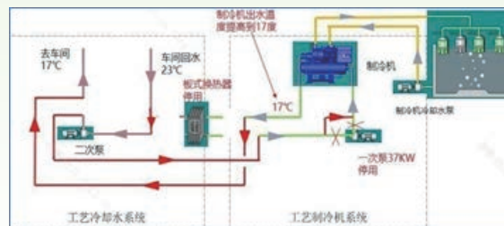
冷卻水系統改造示意圖
