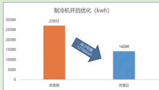
製冷機優化效果
