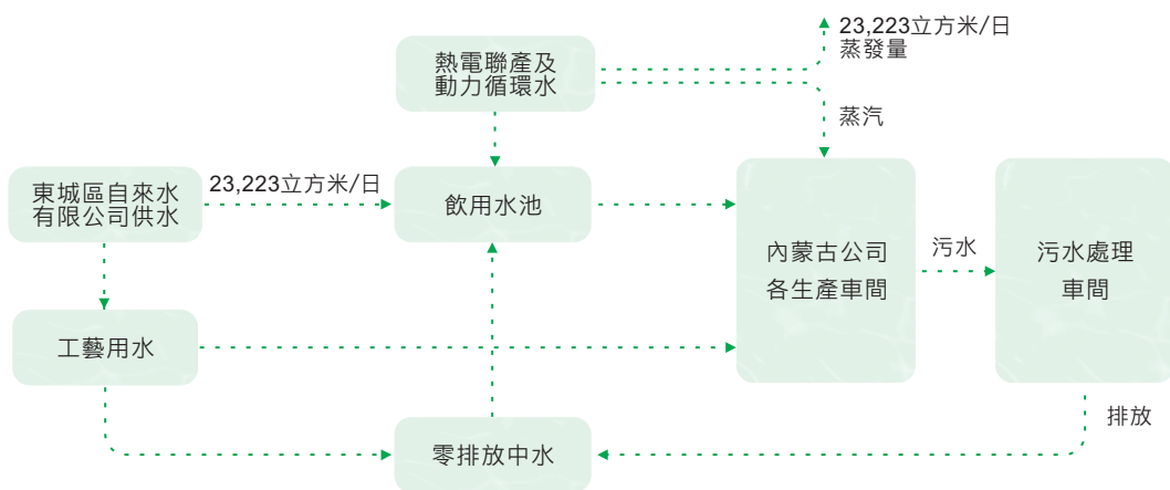
水平衡圖
