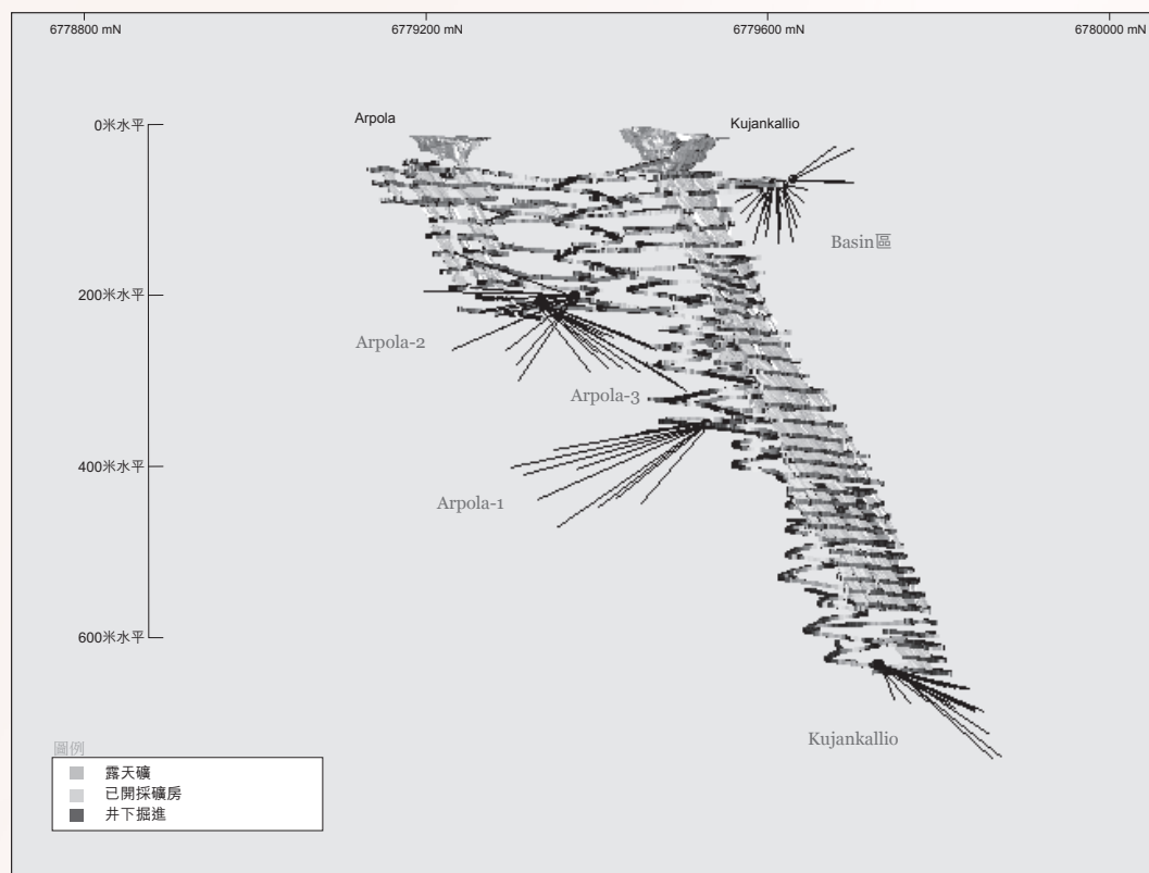
Jokisivu金礦2023年鑽孔活動。向西俯視圖
