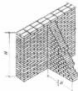
图 F506-2 斜槎
