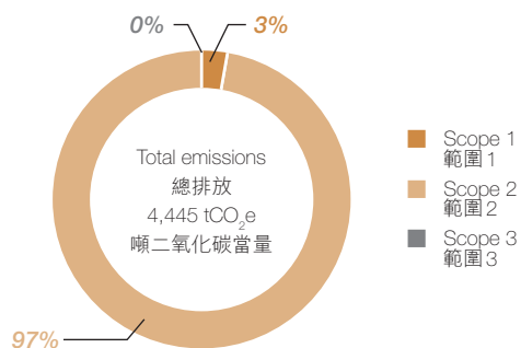
GHG Emissions by Scope FY2023/24 (in %) 按範圍劃分的溫室氣體排放 二零二三／二四財年 (以%計)
